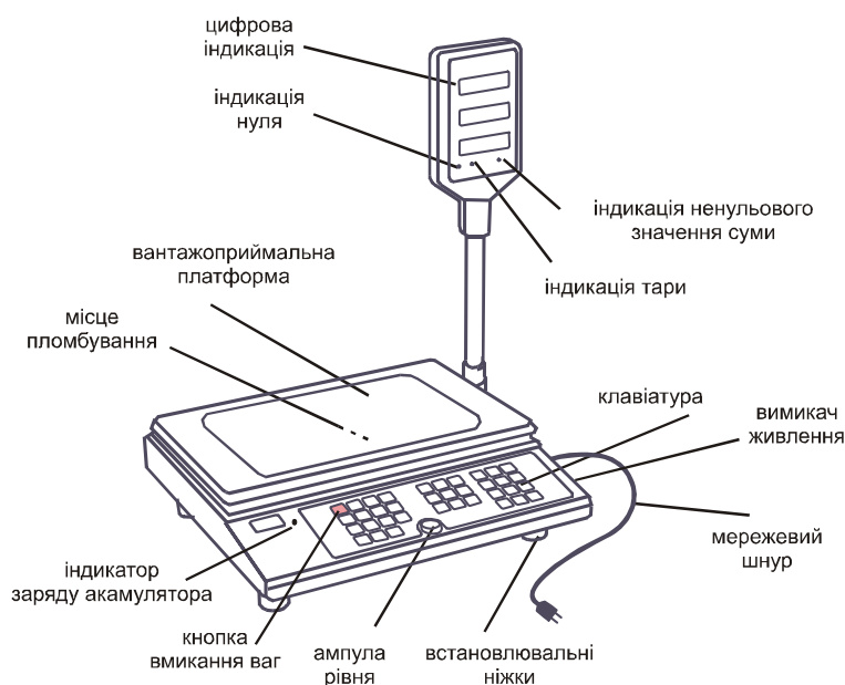
Рис.1. Вигляд ваг
